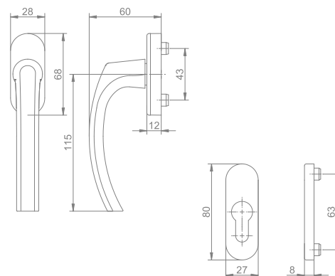
TECHNISCHE ZEICHNUNG
